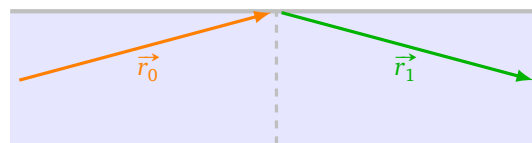
Réflexion totale
