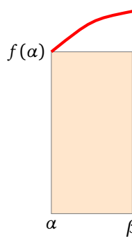
Méthode des rectangles
