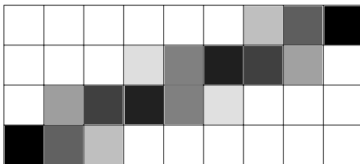
Avec anticrénelage
