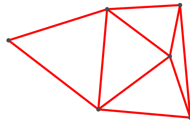
Triangulation de Delaunay
