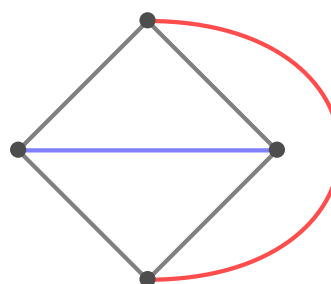
représentation planaire
