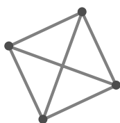
croisement d'arêtes
