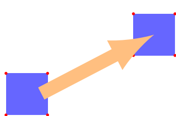
\omega = 0 , pas de vortex
