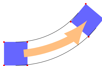
\omega \neq 0
