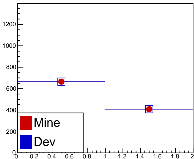
fCaloType
