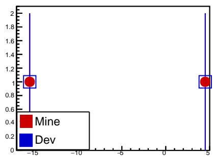
fRho1PtY
