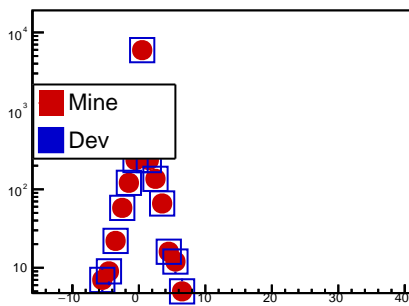
fRho1PtZ
