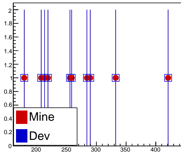
fAmplitude
