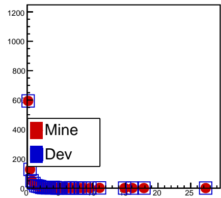
fChi2
