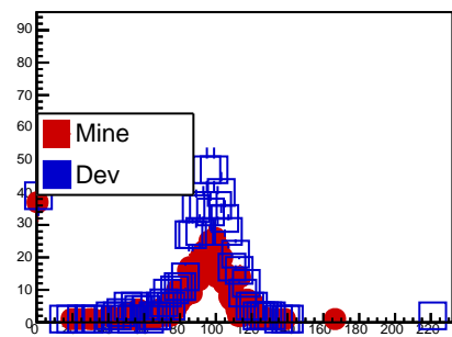
fTPCdEdxTot1R
