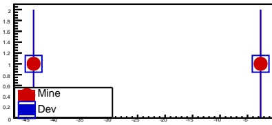
fX
