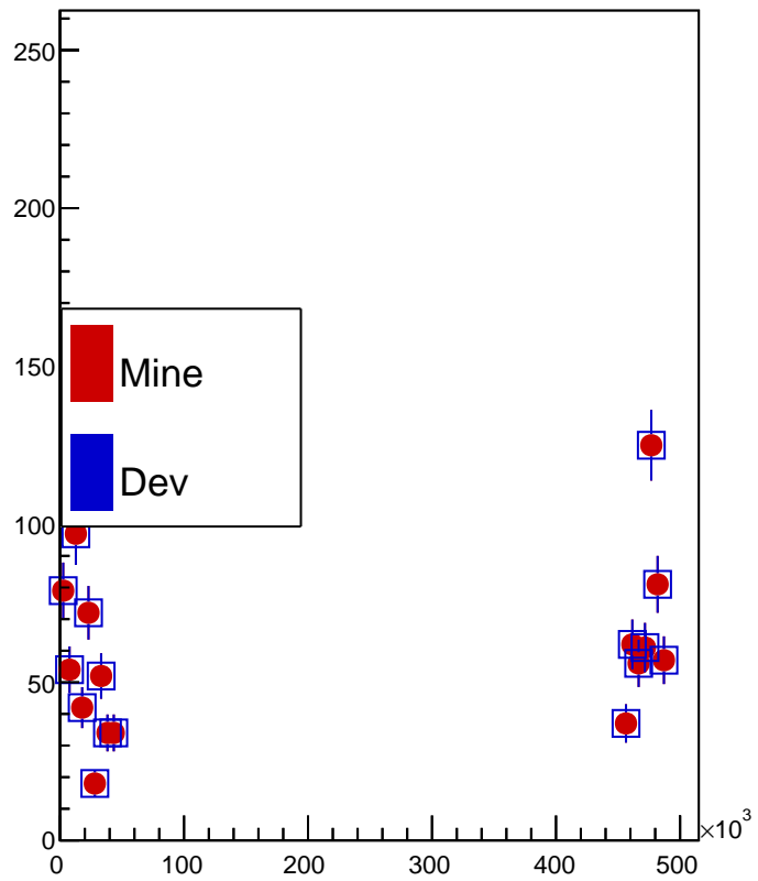
fGlobalBC
