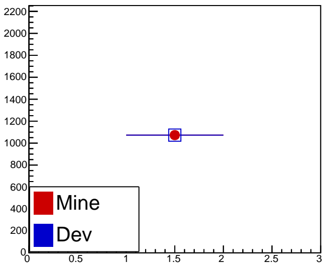
fCellType
