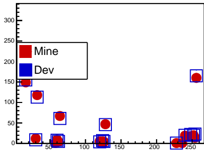
fTPCclusterByteMask
