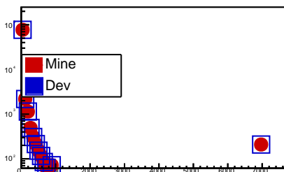
fE
