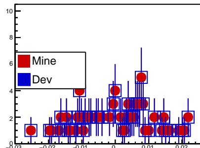
fPosY
