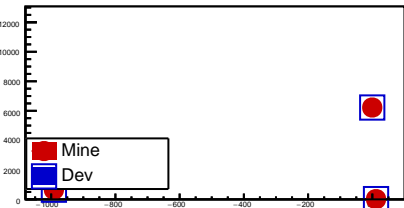
fTPCChi2NCI
