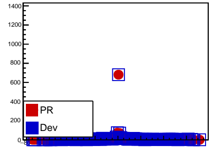
fRho1PtX
