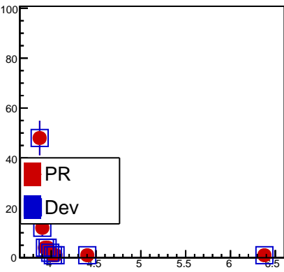
fH4Lmass
