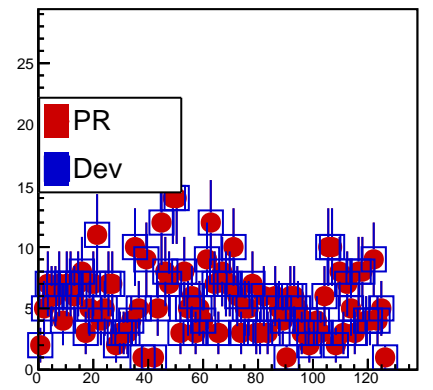
fHMPIDYMip
