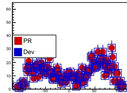
fRhoTglY
