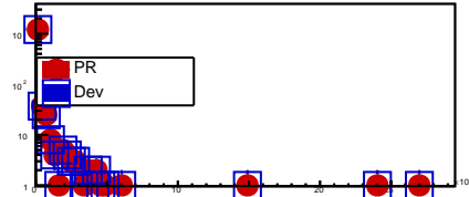
fChi2
