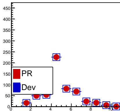
fHMPIDClusSize
