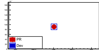
fTRDCh2
