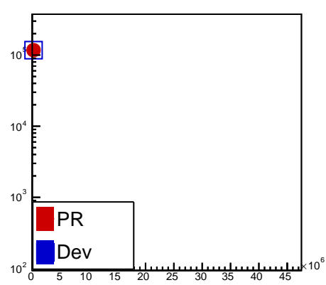
fChi2
