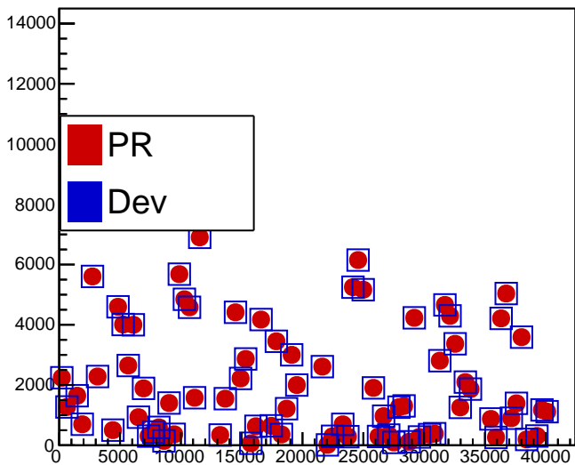
fIndexBCs
