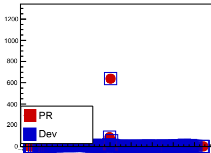
fRho1PtY
