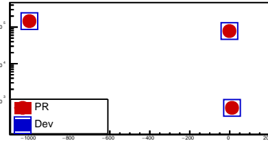
fTRDExpMom
