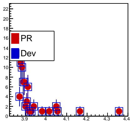
fH4Lmass
