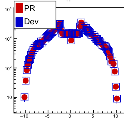
fY
