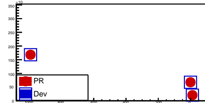
fTOFCh2
