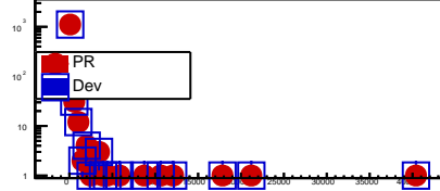
fMatchScoreMCHMFT
