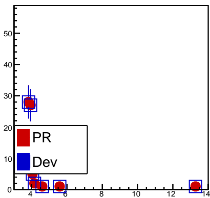
fH4Lmass
