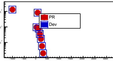
fTPCSignal
