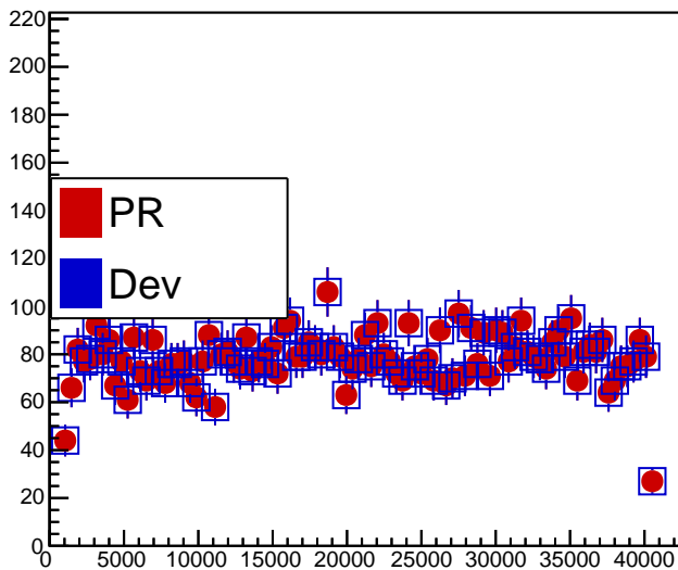
fIndexBCs
