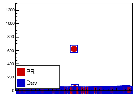
fRho1PtTgl
