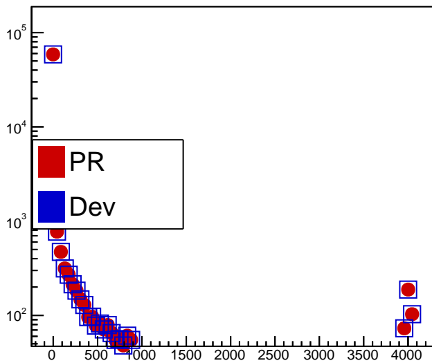
fChargeC
