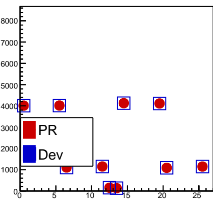
fChannelT
