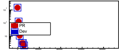
fMatchScoreMCHMFT
