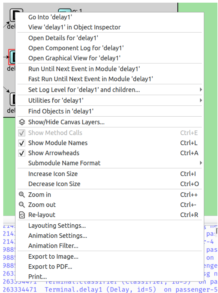
Fig. 7.14: Submodule context menu
